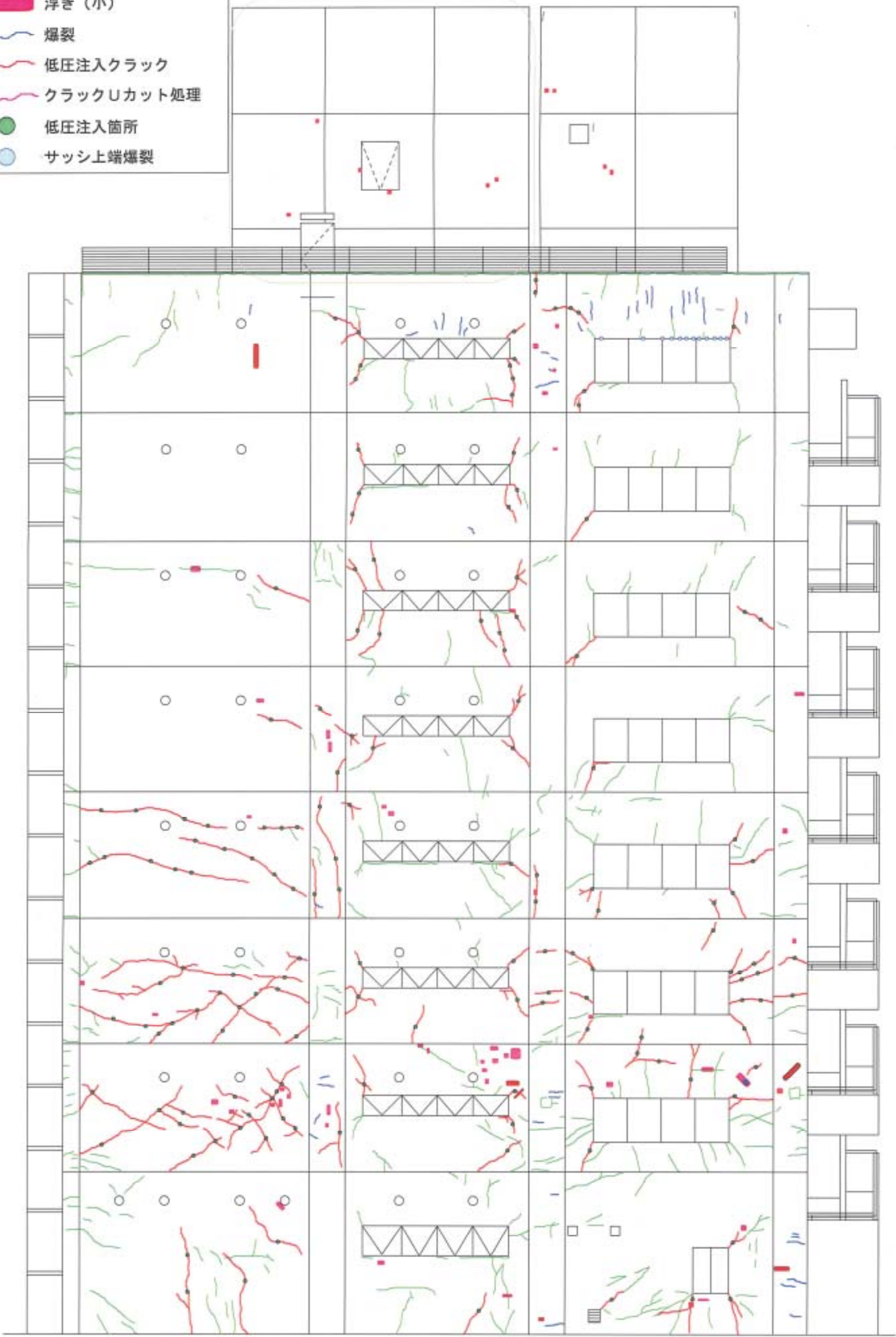
北立面図
