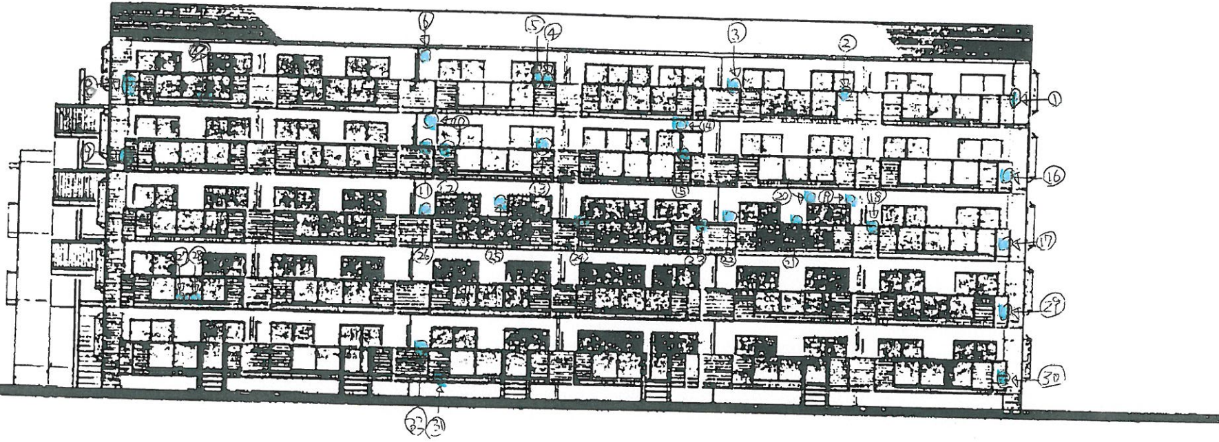
南東立面図
