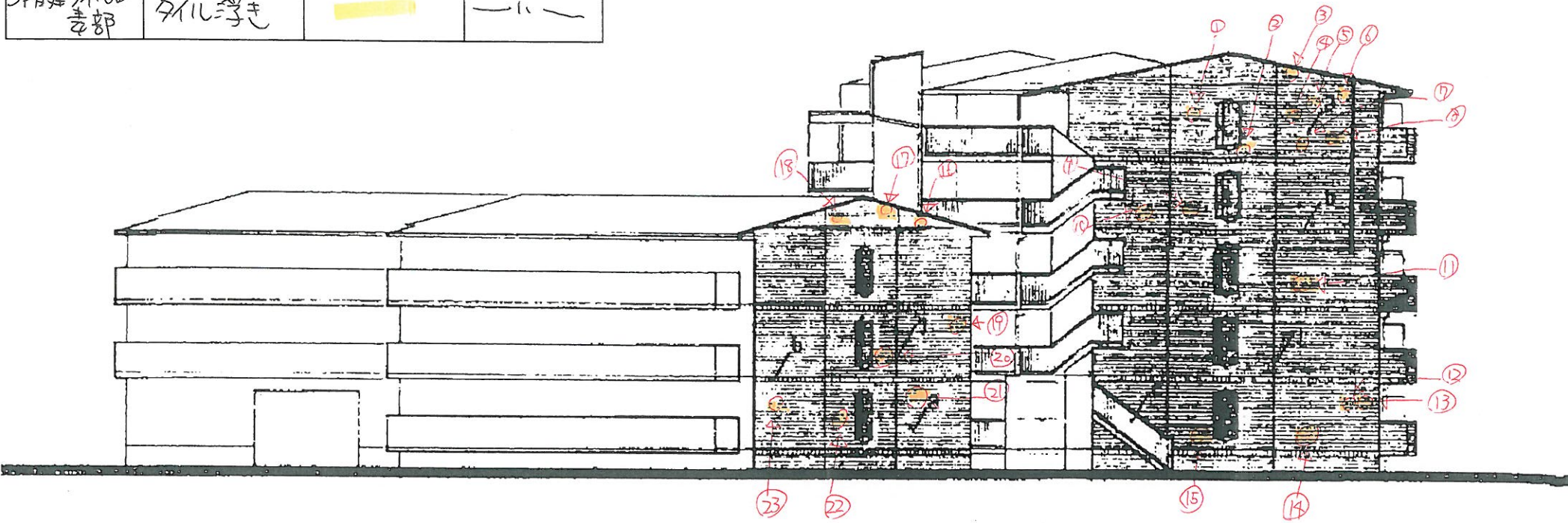
南西立面図
