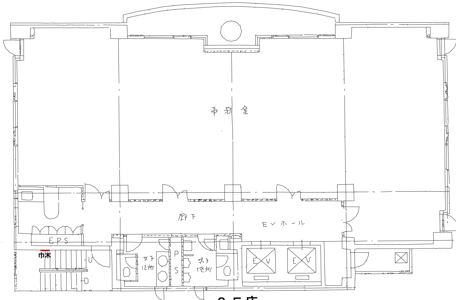
8 F 床
